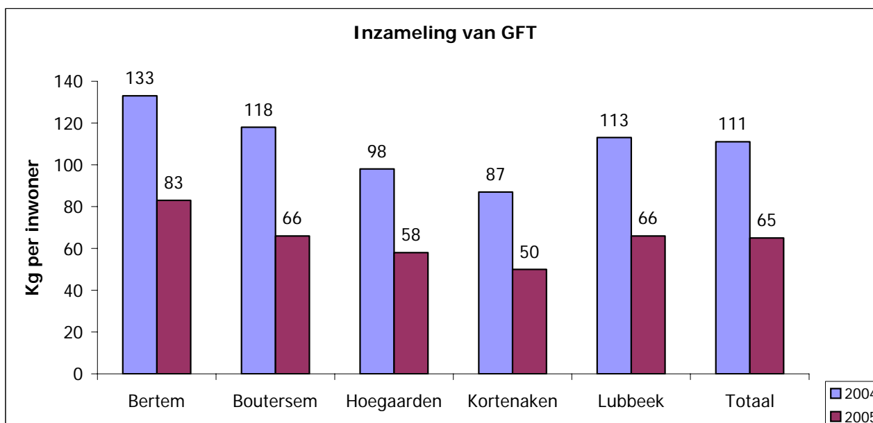
Grafiek 2: Inzameling van GFT in de 5 DifTar-gemeenten
